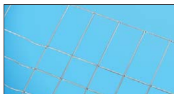
Art. TM 4531 el. svařovaná zinkovaná kari síť (oka 50 x 50 mm x 2 mm drát)
