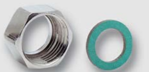
Art. Y434xx matice TFA včetně těsnění KLINGERSIL (250°C)
