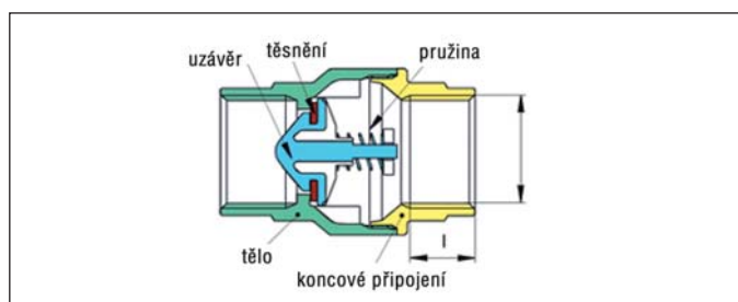
Art. Y388x univerzální zpětná klapka EUROBLOCK se zvětšeným průtokem o 33% ISO 7, T = -20° – 100°C, PN 40 (těsnění pryž NBR)
